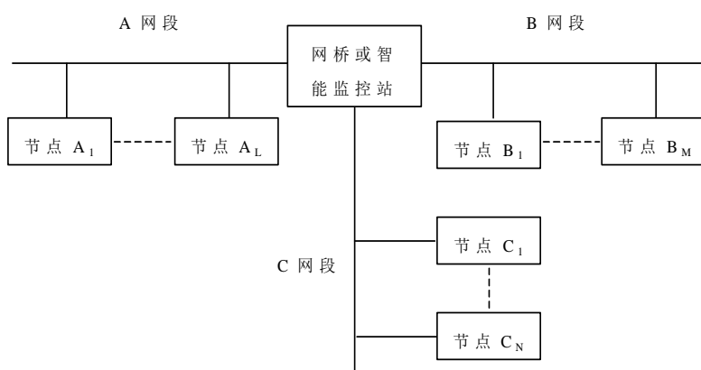
图 5 分段法
