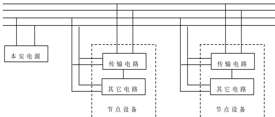
图 7 统一供电法
