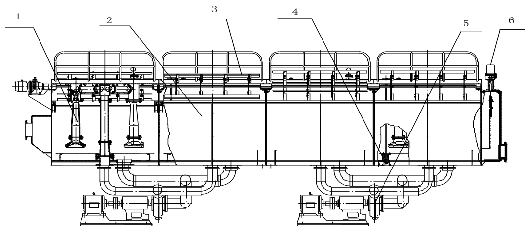
1 充气搅拌装置 2 槽箱 3 刮泡机构 4 放矿装置 5 渣浆泵 6 液面调整机构
