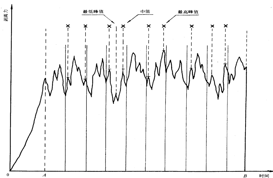
图C.1 剥离曲线处理示意图
