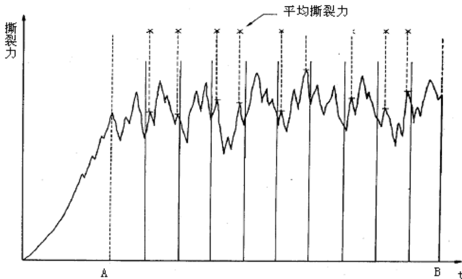
图D.4 撕裂力曲线处理示意图
