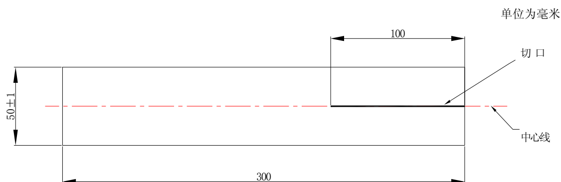
图D.1 撕裂试验用试件示意图
