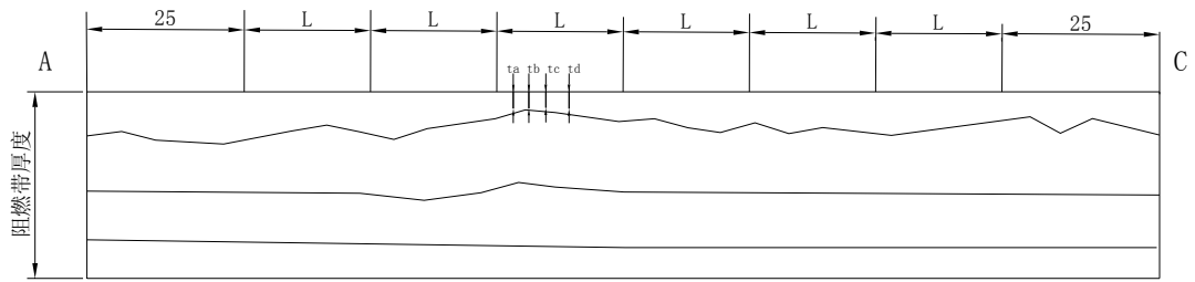
图 A.3 测定覆盖层厚度
