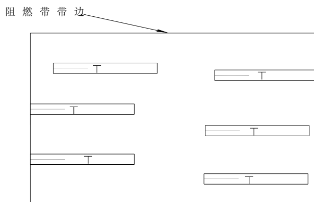
图D.2 试件切割位置及标记
