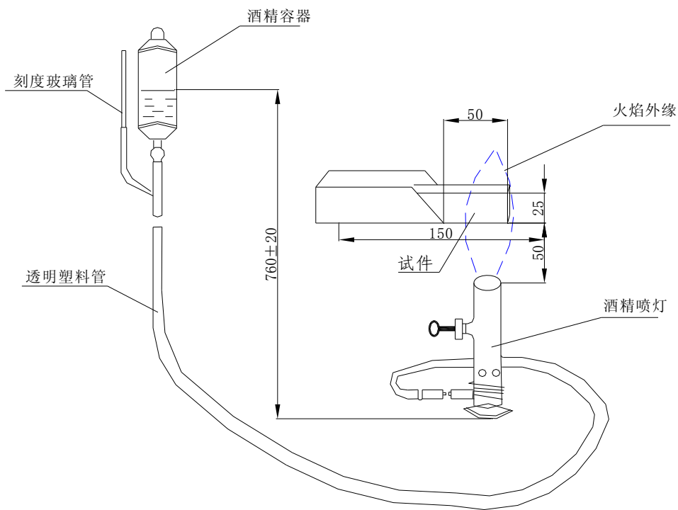
图 G.3 试件燃烧位置示意图
