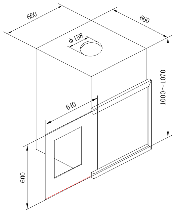
图 G.1 燃烧试验箱示意图
