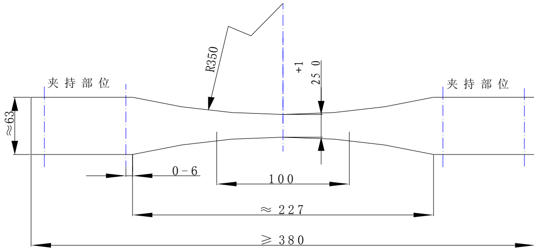
A型试样
