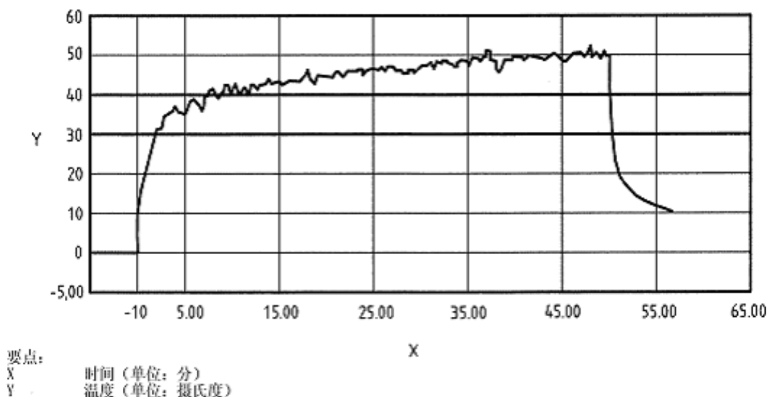
图H.5 典型排气温度校准曲线
