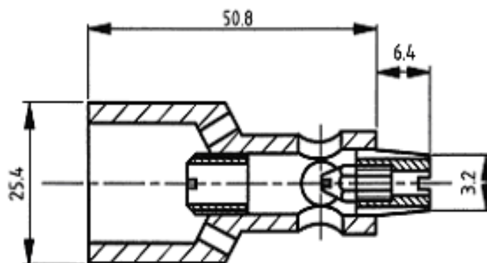
图H.4 丙烷燃烧器的喷射头
