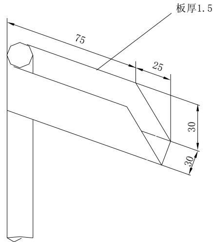
图G.2 酒精喷灯燃烧试验支架示意图
