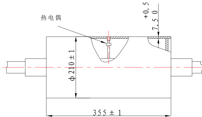
图F.1 钢滚筒示意图
