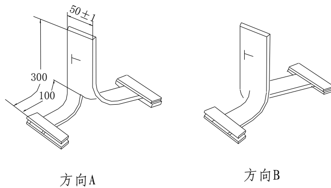
图D.3 撕裂试验安装方式
