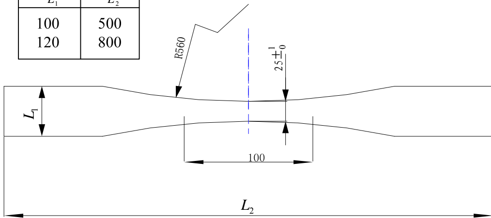
B型试样
