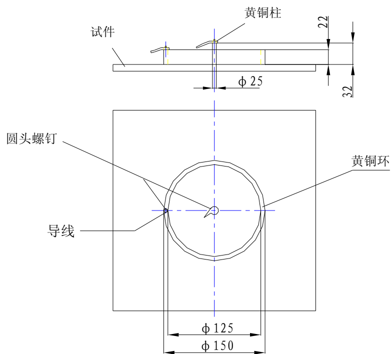
图 E.2 电极尺寸示意图
