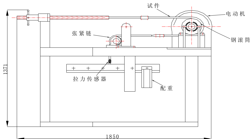
图F.2 滚筒摩擦试验台示意图
