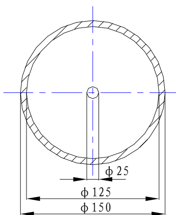
图 E.1 涂胶示意图
