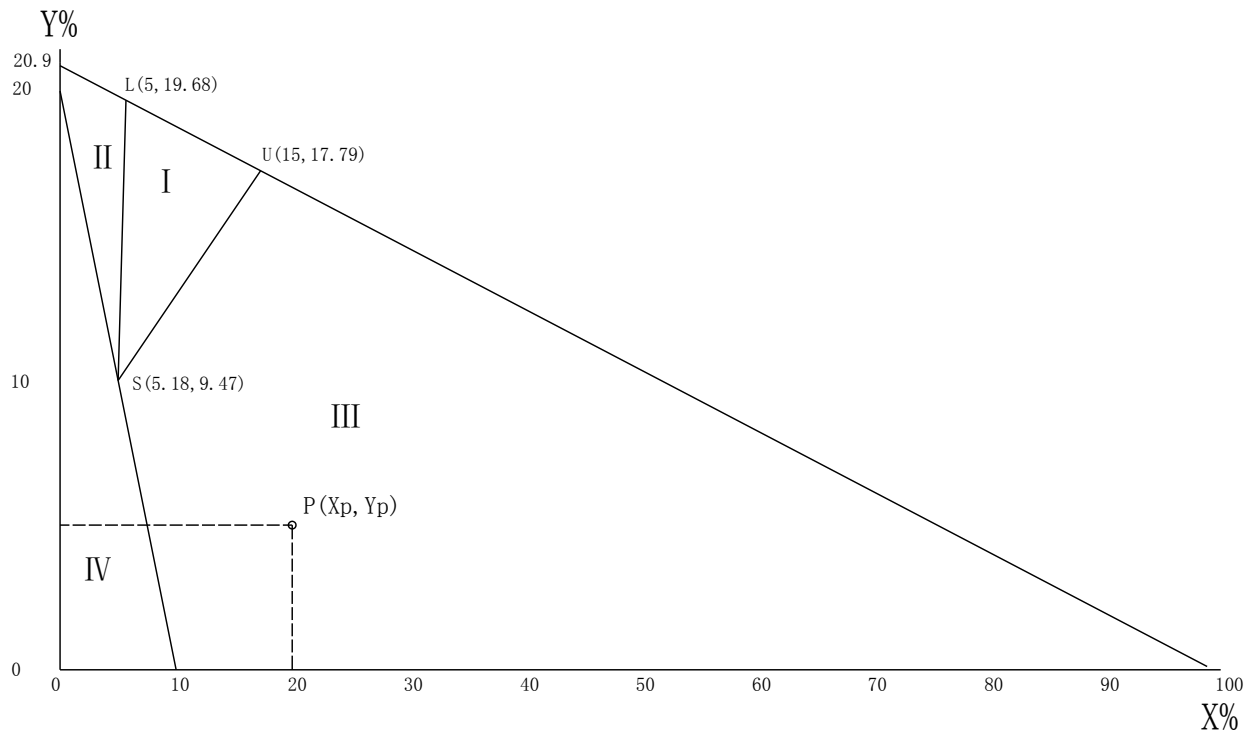
图 B-1 爆炸三角形图
