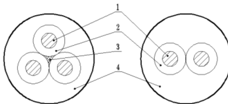
1-导体；2-绝缘；3-填充；4-护套
