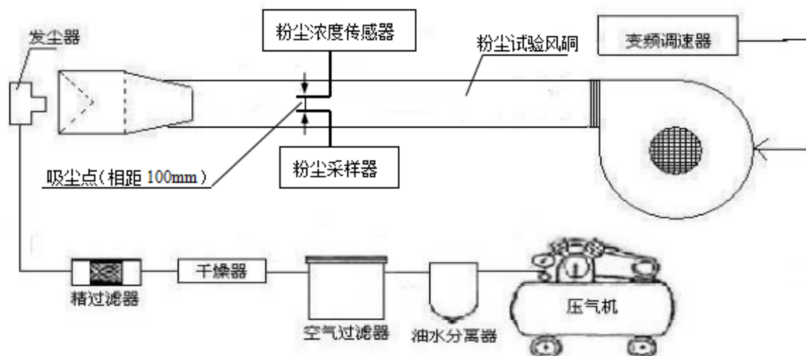
图1 粉尘试验风洞实验系统
