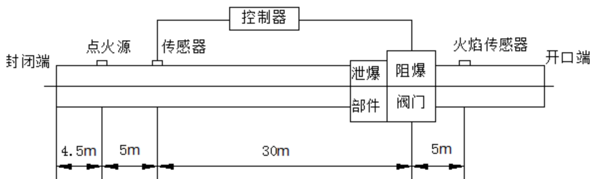
图 1 试验装置示意图
