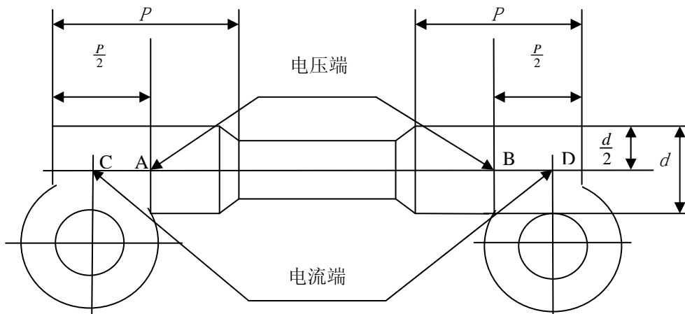
图1 测定单根连线导线接触电阻位置图
