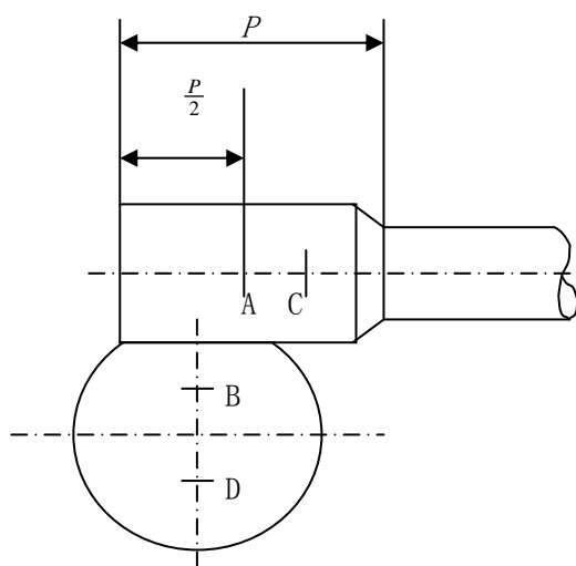
图2 测定连接导线与蓄电池极柱接触电阻位置图
