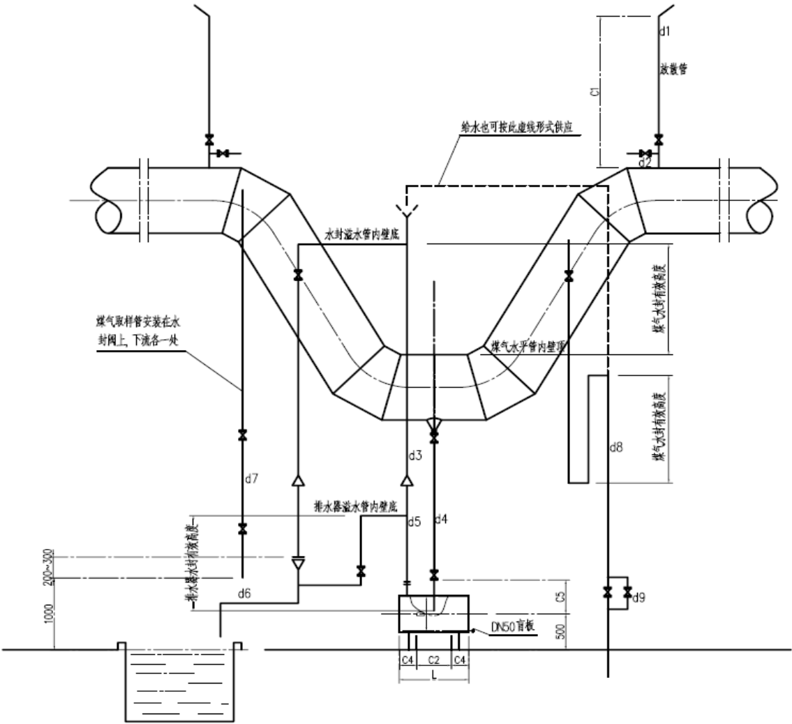
图 A.1 煤气水封管道及附属设备
