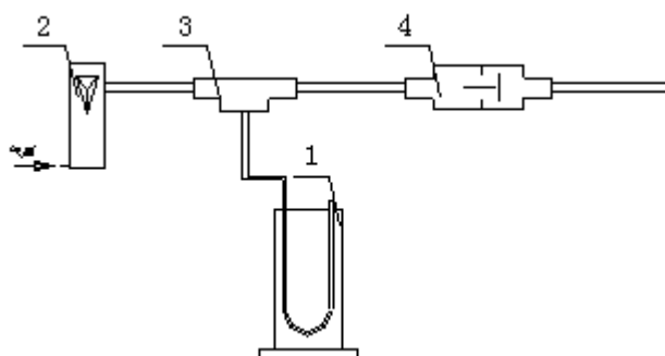
1—水柱压力计（0~1200Pa，分度值10Pa）；2—转子流量计（2.5级）；3—三通管；4—呼或吸气阀。
