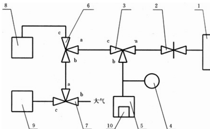
1—高压甲烷瓶；2—减压阀；3、6、7—高压三通阀；4—压力表；5—煤样罐；8—瓦斯解吸仪；9—真空泵；10—煤样杯；a、b、c—三通阀的三个通路
