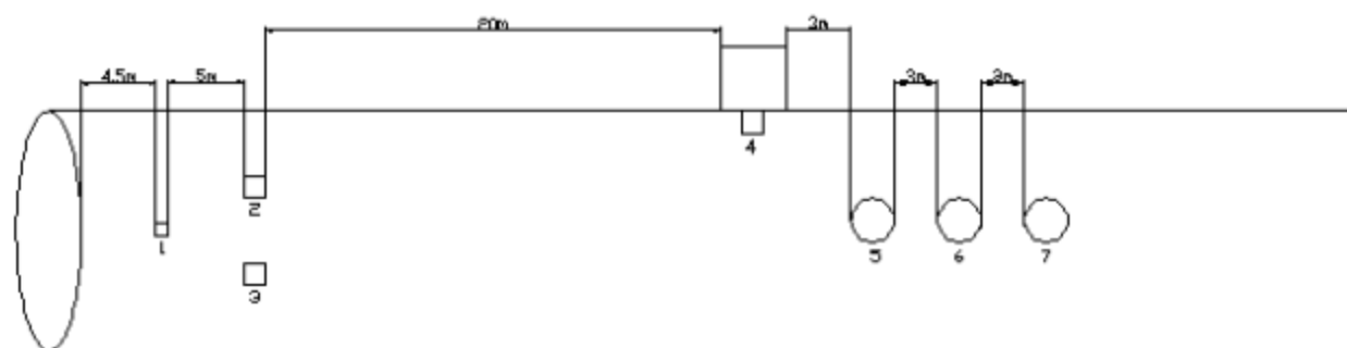
1—点火源 2、3—自动喷粉抑爆装置传感器 4—抑爆器 5、6、7—测试用火焰传感器
