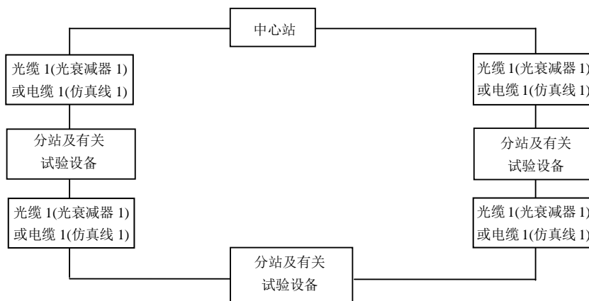
图 2 环形系统设备连接
