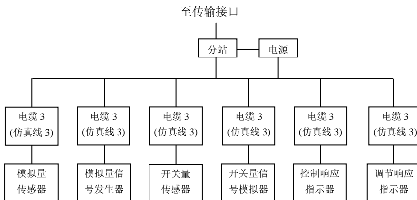
图4 分站设备连接
