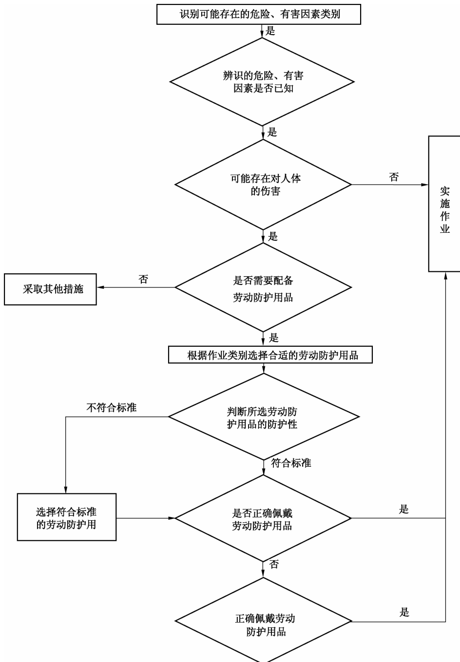
图 1 劳动防护用品的选用程序
