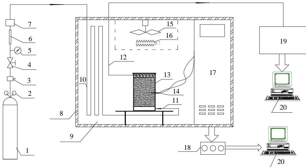
1-干空气瓶；2-减压阀；3-稳压阀；4-稳流阀；5-压力表；6-气阻；7-流量传感器；8-隔热层；9-控温箱； 10-气体预热铜管；11-进气管；12-出气管；13-煤样罐；14-铂电阻温度传感器；15-风扇；16-加热器； 17-控制器及显示键盘；18-数据采集系统；19-气相色谱仪；20-计算机
