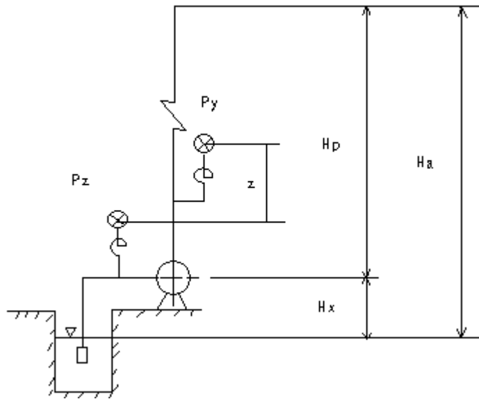
图1 水泵扬程测试布置图
