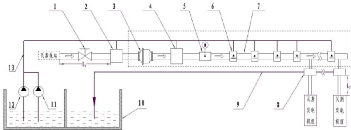
1、截止阀 2、湿式阻火泄爆装置 3、煤矿瓦斯输送管道阻火器 4、泄压溢流阀 5、控制阀门 6、水雾发生器 7、瓦斯输送管道 8、脱水器 9、回水管道 10、水池 11、备用水泵 12、主水泵 13、给水管道
