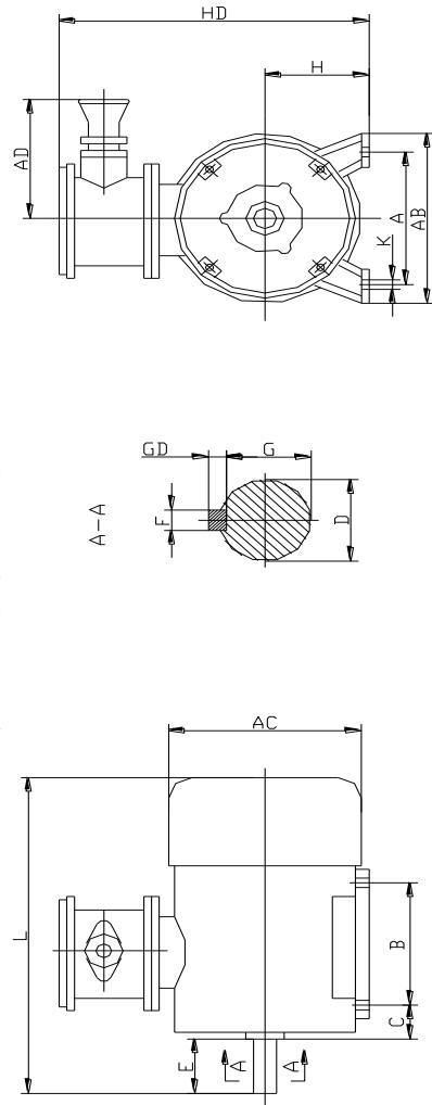
附录 A (资料性附录) 泵用隔爆型三相异步电动机安装尺寸及公差
