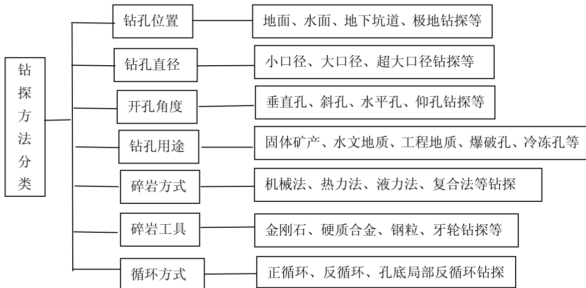
图 1 钻探方法分类示意
