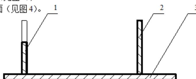
1——焊筋板；2——隔水圈板；3——环形底板。
