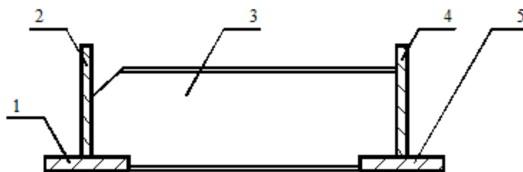
1—内环形底板；2—焊筋板；3—连接工字钢；4—隔水圈板；5—外环形底板。
