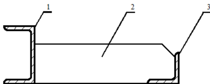
1—内缘槽钢；2—连接加劲板；3—外缘角钢。
