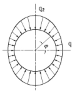
图1 不均匀荷载变化规律图
