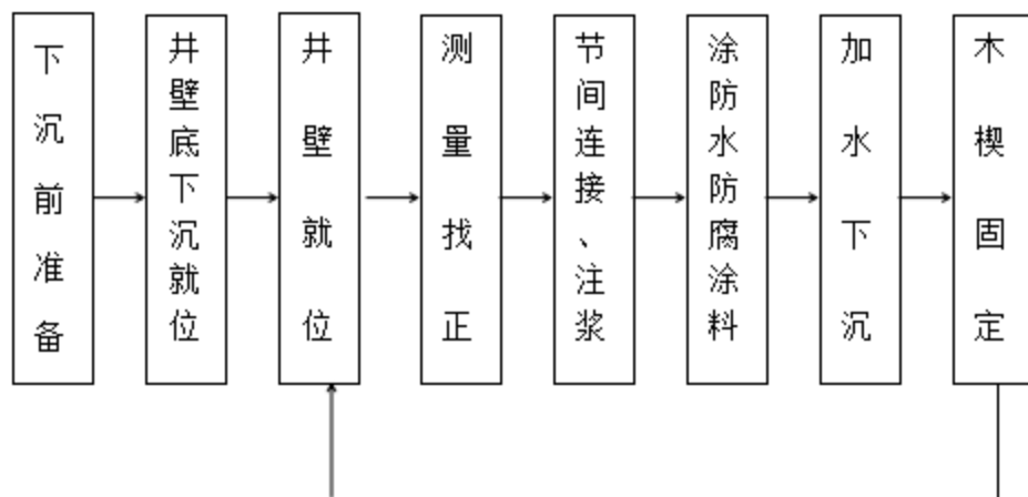
图5 井壁悬浮下沉工艺流程示意图
