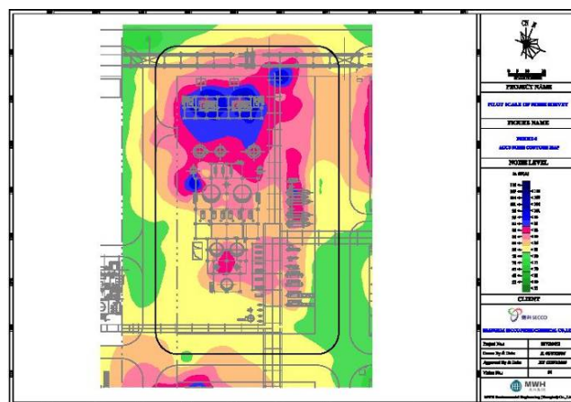
图 A. 22 噪音图谱
