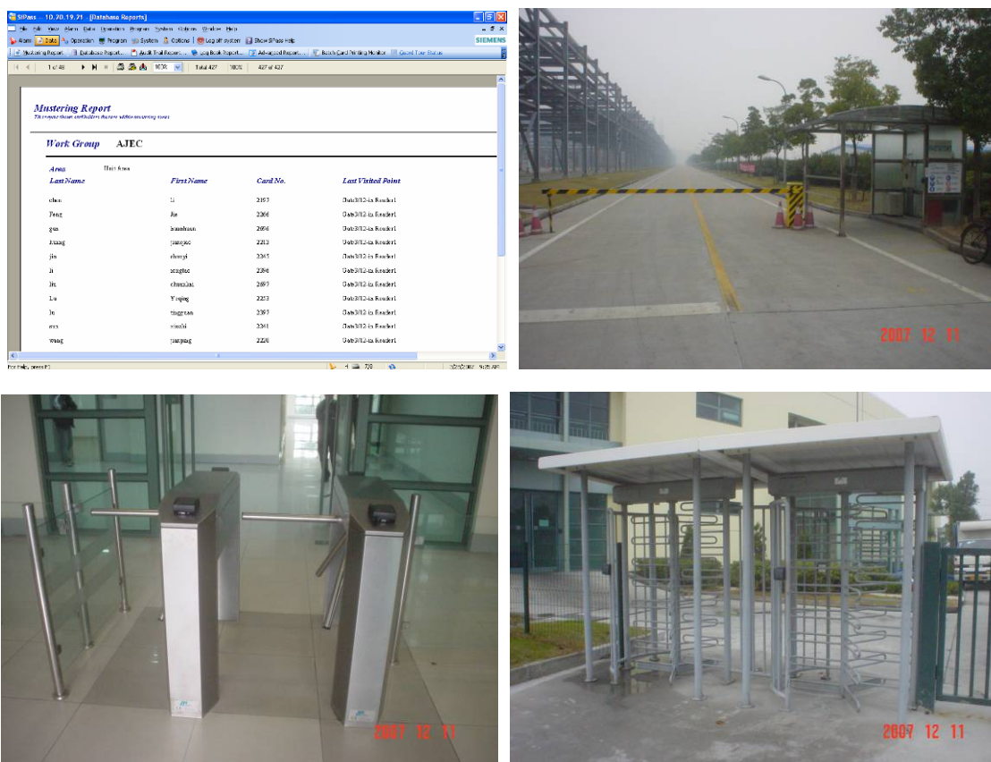
图 A.28 门禁管理系统
