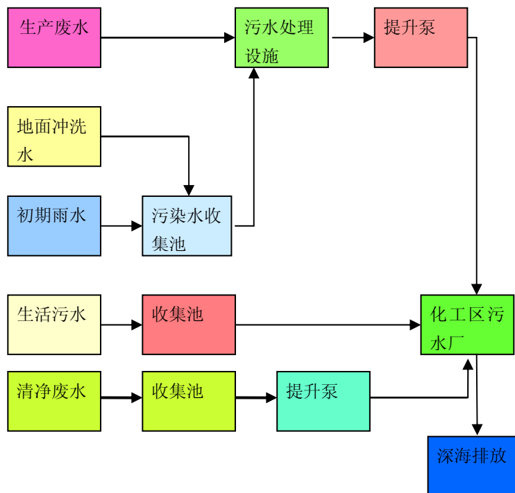
图 A. 23 废水分类示意图
