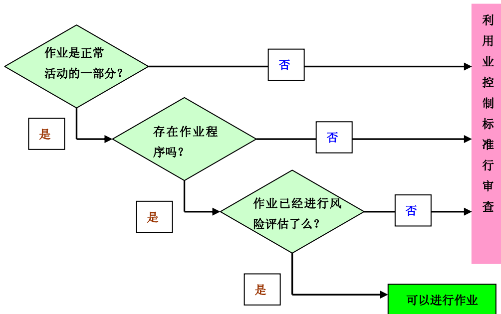
图 A.19 作业许可判断流程
