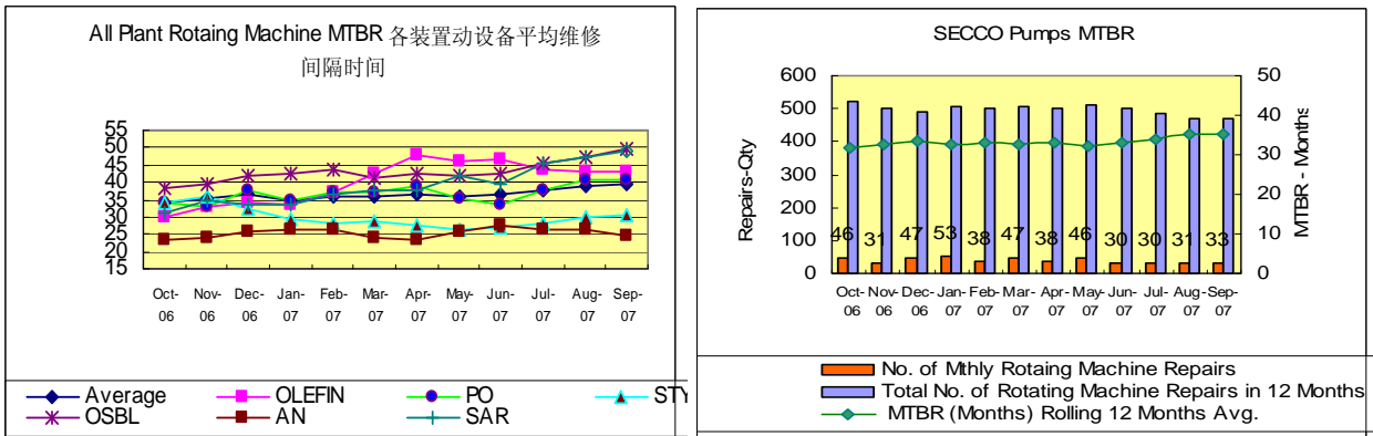
图 A. 14 动设备平均维修间隔时间
